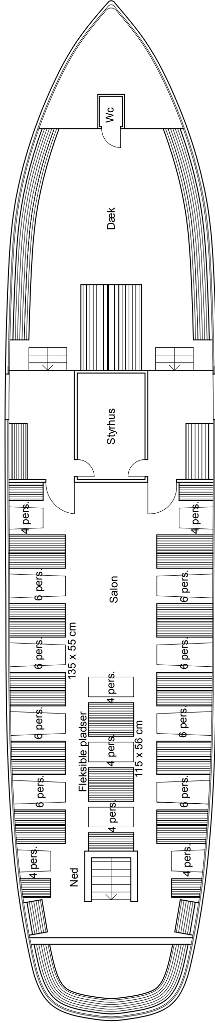
Hejren 1:100
