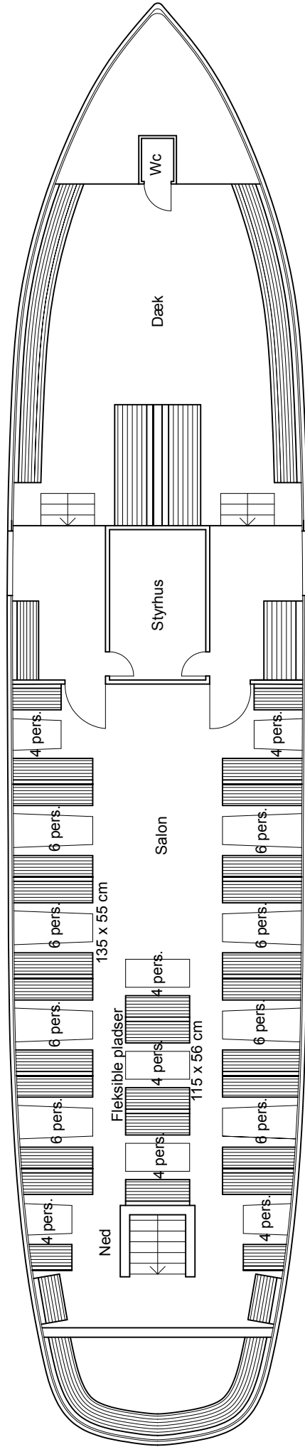
Hejren 1:100
